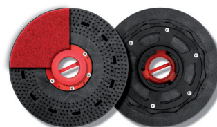
Plateau Padloc support disque Ø406mm réf.606401
